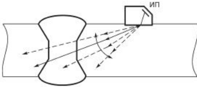
Рисунок 21 - Способ сканирования качающимся лучом
