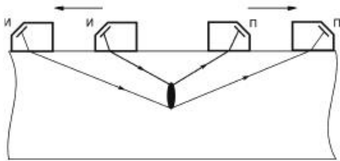
Рисунок 5 - Дифракционный
