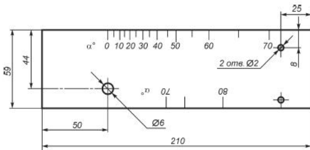
Рисунок А.1 - Эскиз меры СО-2
