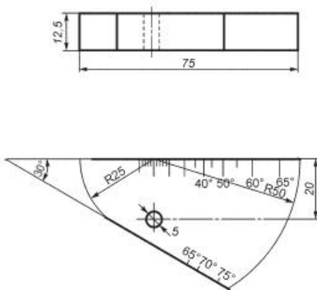
Рисунок Б.3 - Эскиз НО V2
