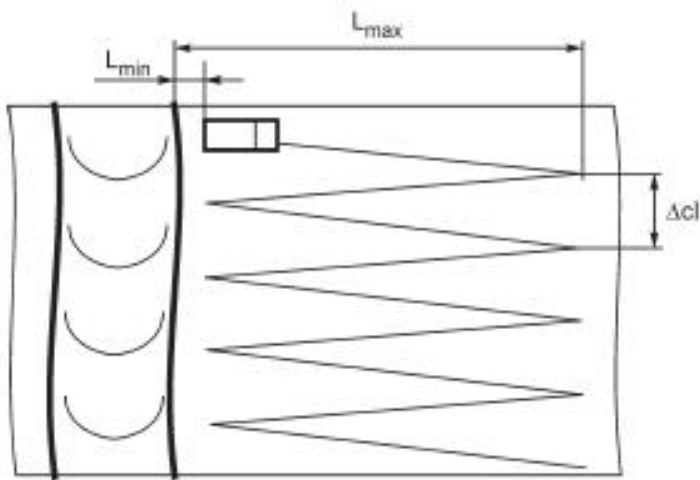
Рисунок 19 - Варианты способа поперечно-продольного сканирования
