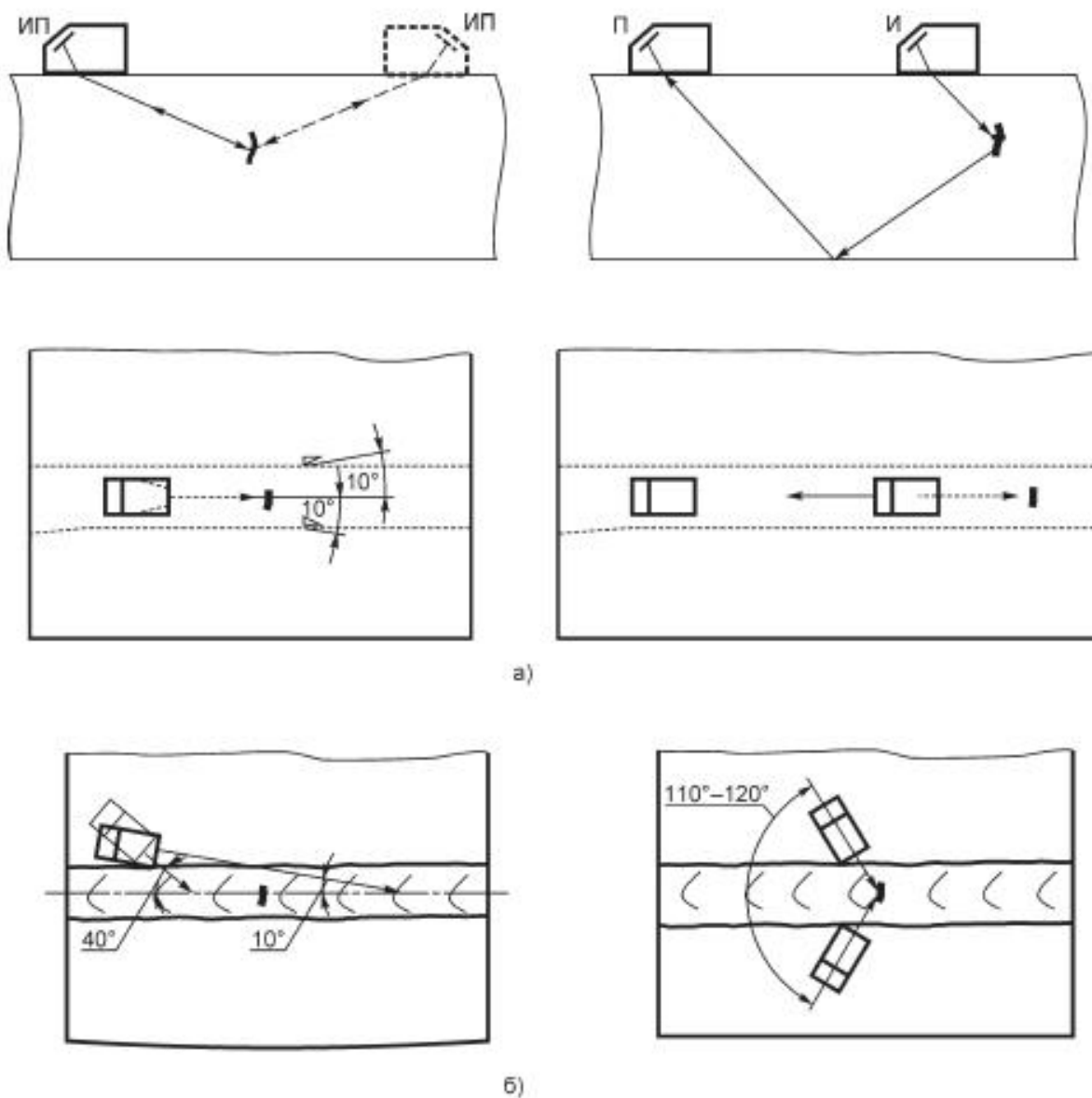
Рисунок 17 - Схема прозвучивания стыковых сварных соединений при контроле для поиска поперечных трещин: а) - со снятым валиком шва; б) - с удаленным валиком шва
