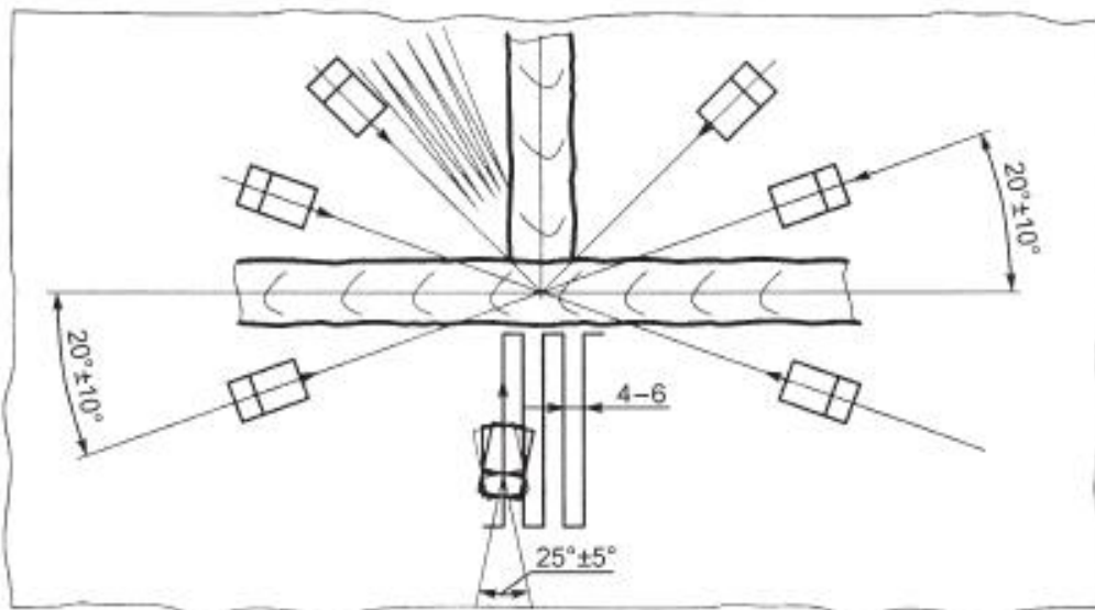
Рисунок 18 - Схемы прозвучивания мест пересечений стыковых сварных соединений
