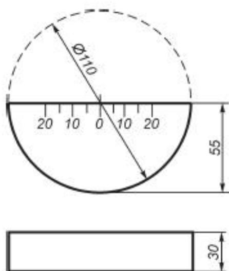
Рисунок А.2 - Эскиз меры СО-3
