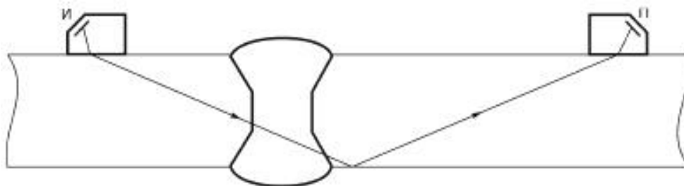
Рисунок 2 - Зеркально-теневого
