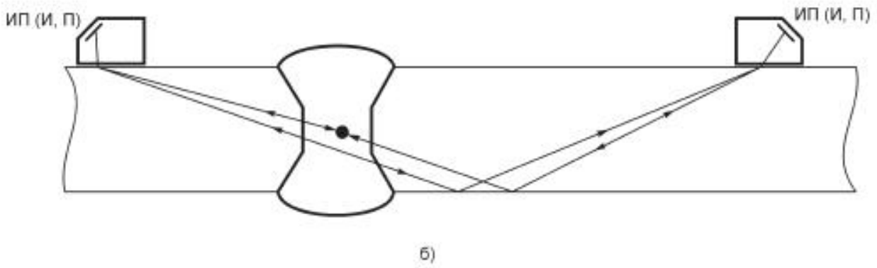
Рисунок 3 - Эхо-теновой прямым (а) и наклонными (б) ПЭП
