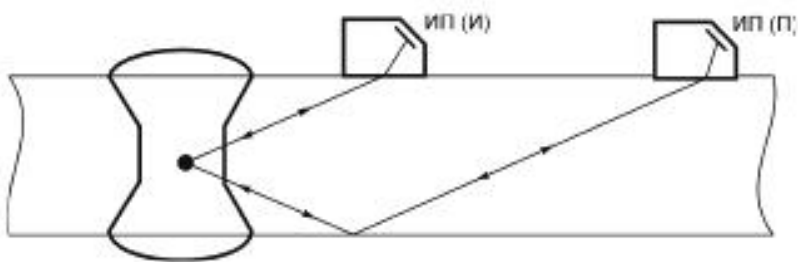
Рисунок 4 - Эхо-зеркальный
