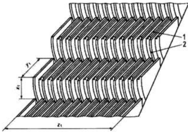
Рисунок 3 - Ступени (основные размеры)
