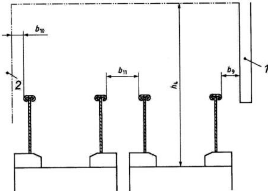
Рисунок 4 - Расстояния между элементами конструкции здания и эскалатором
