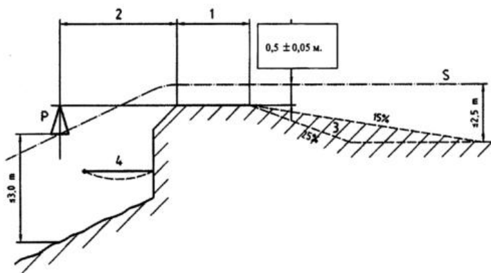
Рисунок 2. Зоны высадки КД с креслами
