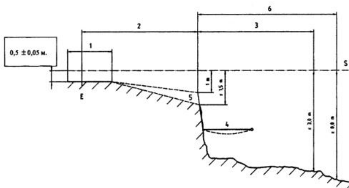
Рисунок 1. Зоны посадки на кресельных КД
