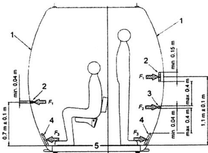
Рисунок 4. Схема расположения защитных элементов
